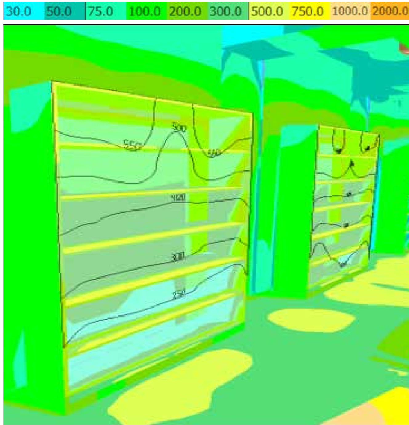
Simulation photométrique
